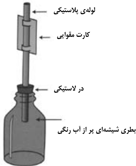
دماسنج دست‌ساز
